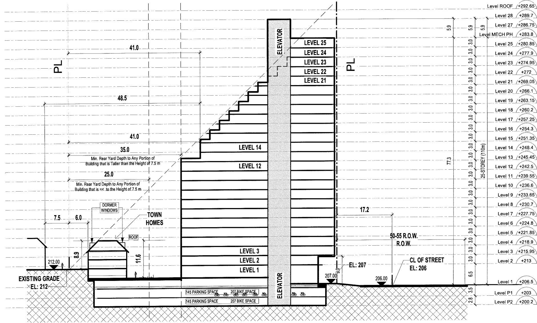
1 Section A 1 : 500
