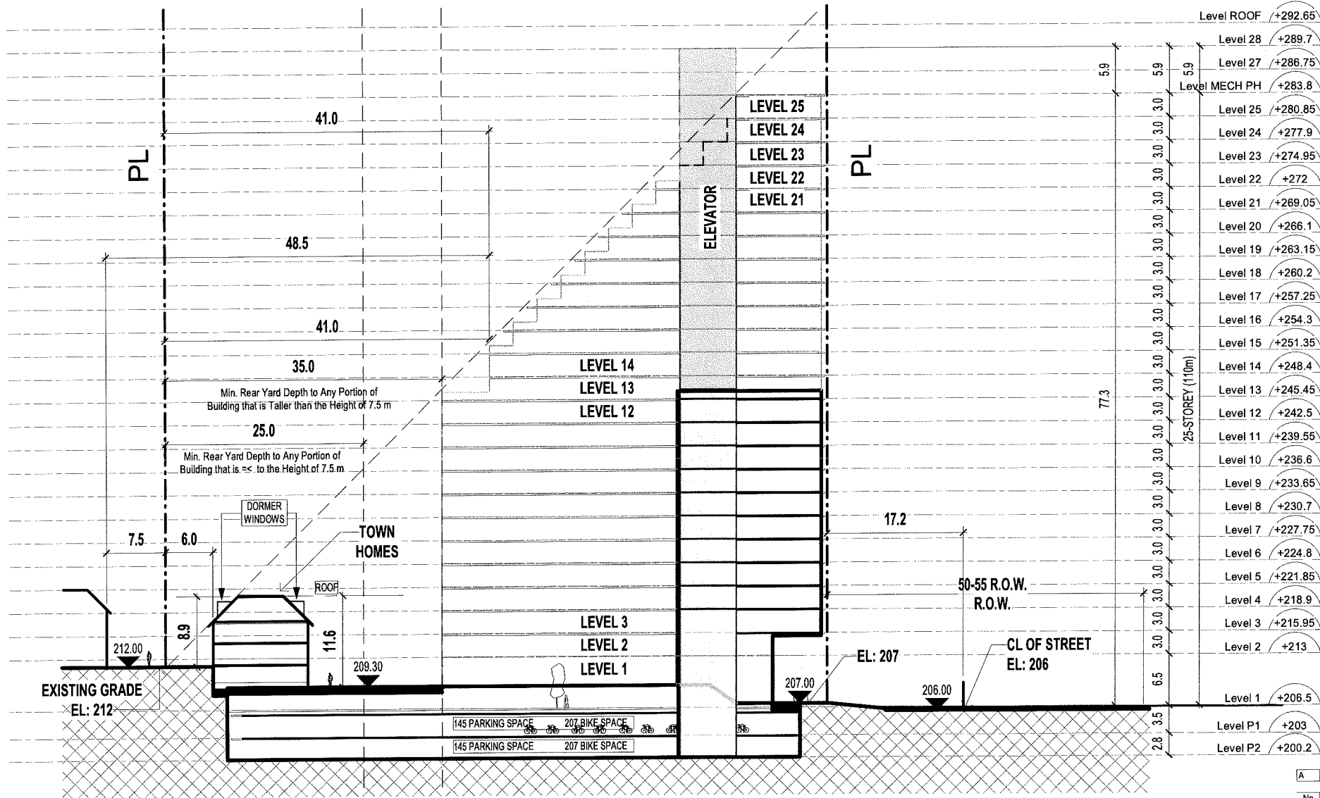
1 Section B 1 : 500
