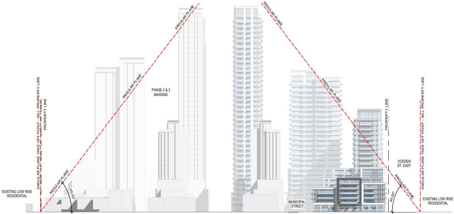
① Hansen Rd. - Phase 2 & 3 1:500
